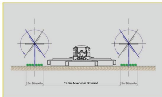
Abb.: Prinzipskizze
